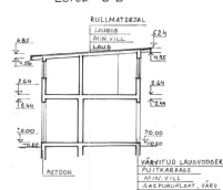
LÖIGE B-B
