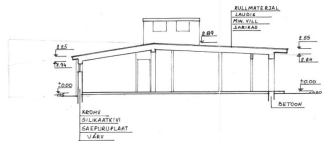
LÕIGE B-B
