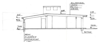
LÕIGE B-B
