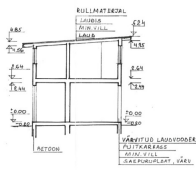
LÕIGE B-B
